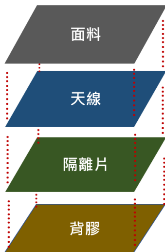
UHF-F06T天線結構示意圖
